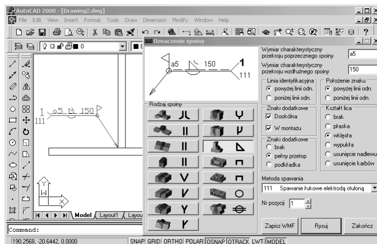
Rysunek 5.2. Okno programu PolSpaw przy pracy w programie AutoCAD
