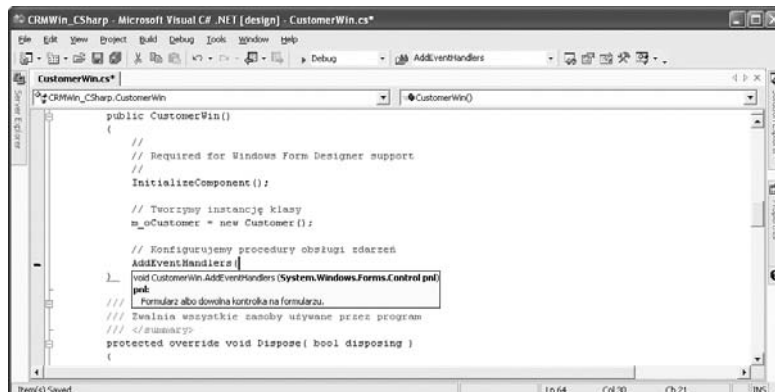
Rysunek 3.5. Funkcja Parameter Info pobiera informacje z elementu <param> w komentarzu XML
