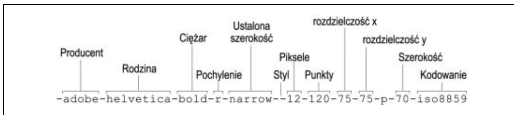
Rysunek 14.2. Pola definicji czcionki
