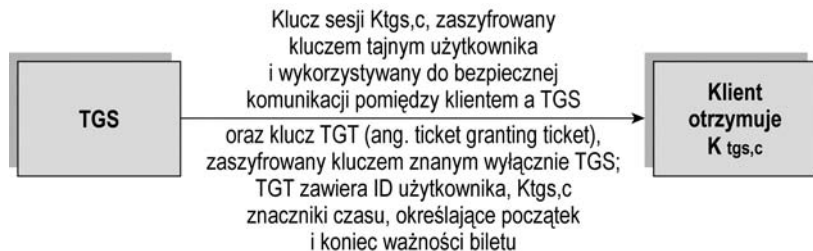
Rysunek 3.2. Wymiana klucza sesji i biletu TGT pomiędzy klientem a TGS
