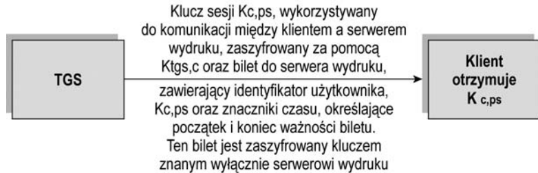
Rysunek 3.4. Transmisja klucza sesji klienta i serwera wydruku
